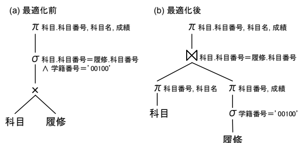
図1 処理木を使った最適化
